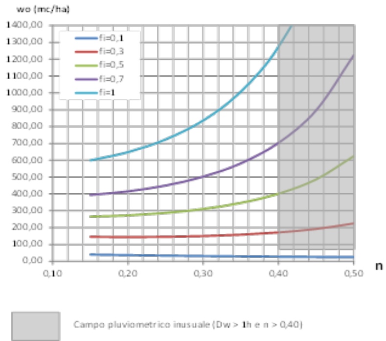
Figura 7 - Grafici della durata D_w (eq. 12») e del volume specifico critico di invaso w_0 (eq. 13») in funzione di n , per \alpha=80 mm/ora e per u = 10 l/s per ettaro \alpha = 80 mm/ora n ; u = 10 l/s per ettaro
