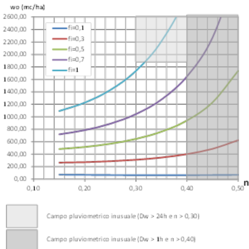
Figura 9 – Grafici della durata D_w (eq. 12») e del volume specifico critico di invaso w_o (eq. 13») in funzione di n , per a=40 mm/ora e per u = 20 l/s per ettaro
