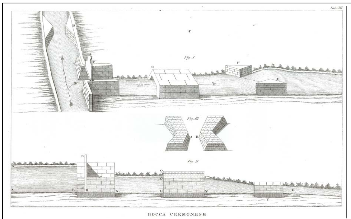
Illustrazione di una bocca irrigua con òpera di misura della portata 'alla cremonese'
