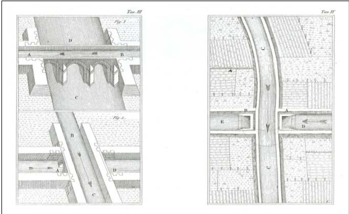
Illustrazione di una bocca irrigua con òpera di misura della portata 'alla cremonese'
